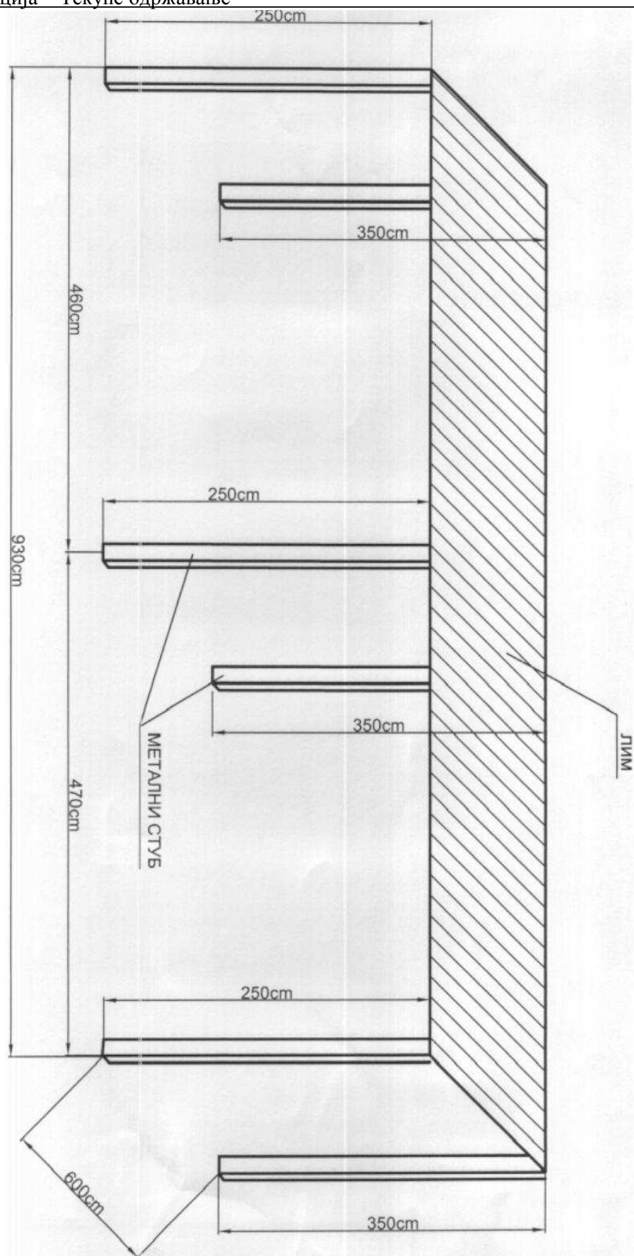
СКИЦА 1 НАДСТРЕШНИЦА
